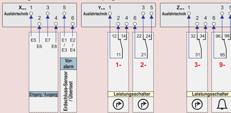
rückseitig montierte Steuerstecker 6 polig
