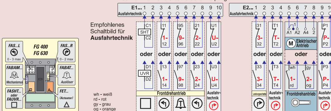
Seitlich montierte Steuerstecker 10 polig
